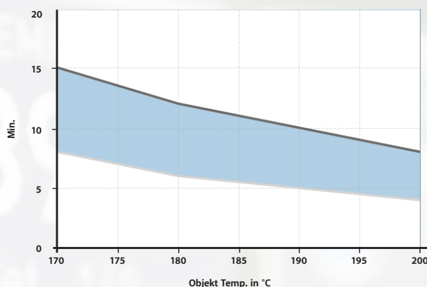
Einbrenndiagramm POLYFLEX® PES-55-NT-DS
